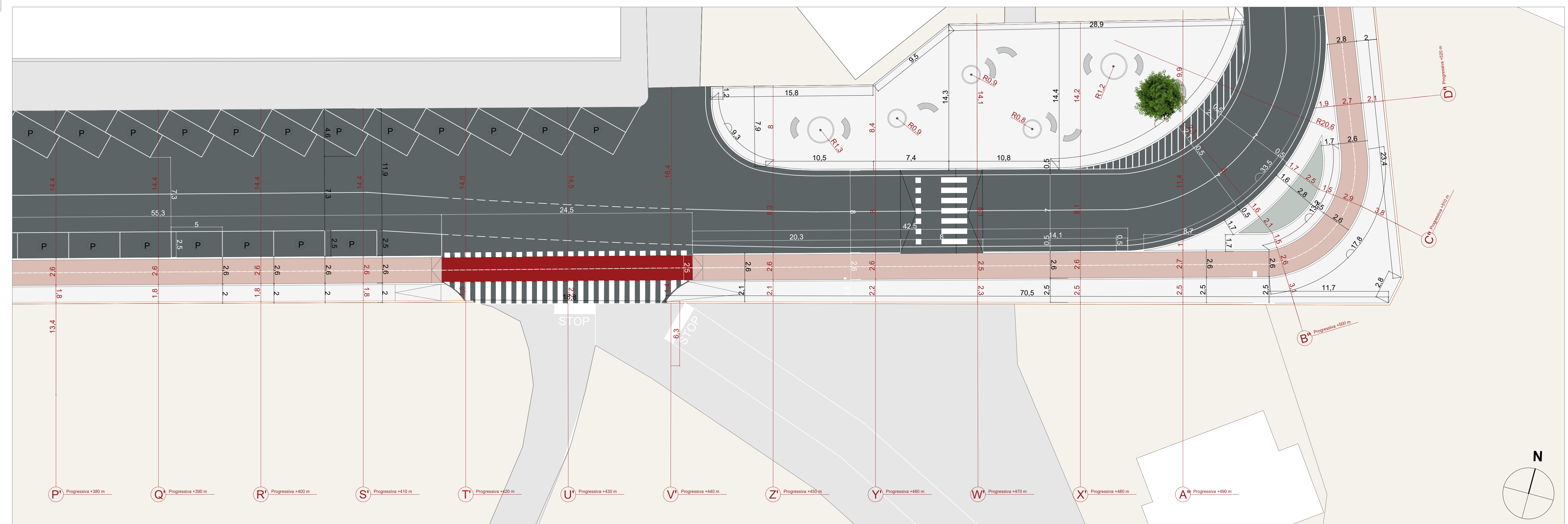
PLANIMETRIA AREA DI INTERVENTO 3 - SCALA 1:200
