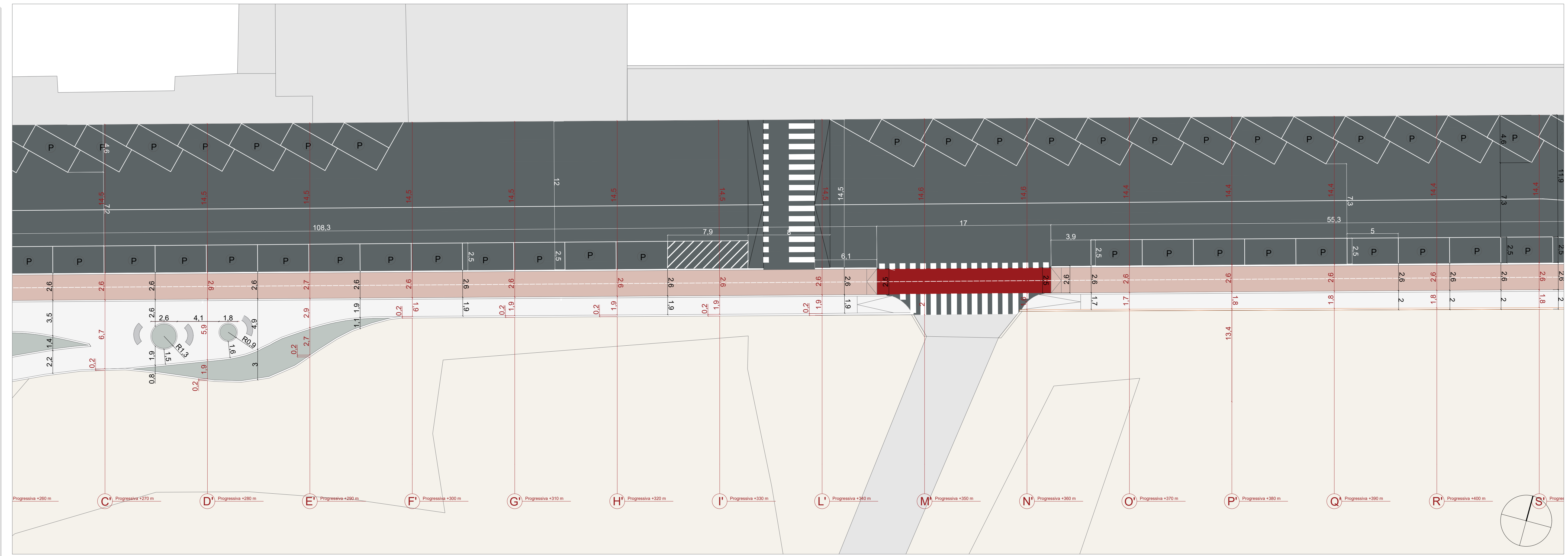
PLANIMETRIA AREA DI INTERVENTO 3 - SCALA 1:200
